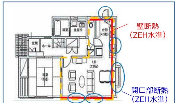
住宅の一区画の断熱改修イメージ図（②の基準に適合）
